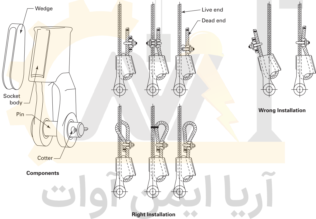
Fig. 26-3.1.1-2 Wedge Sockets
