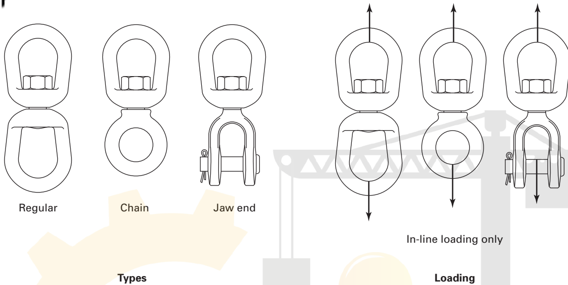
Fig. 26-4.1.1-2 Swivels
