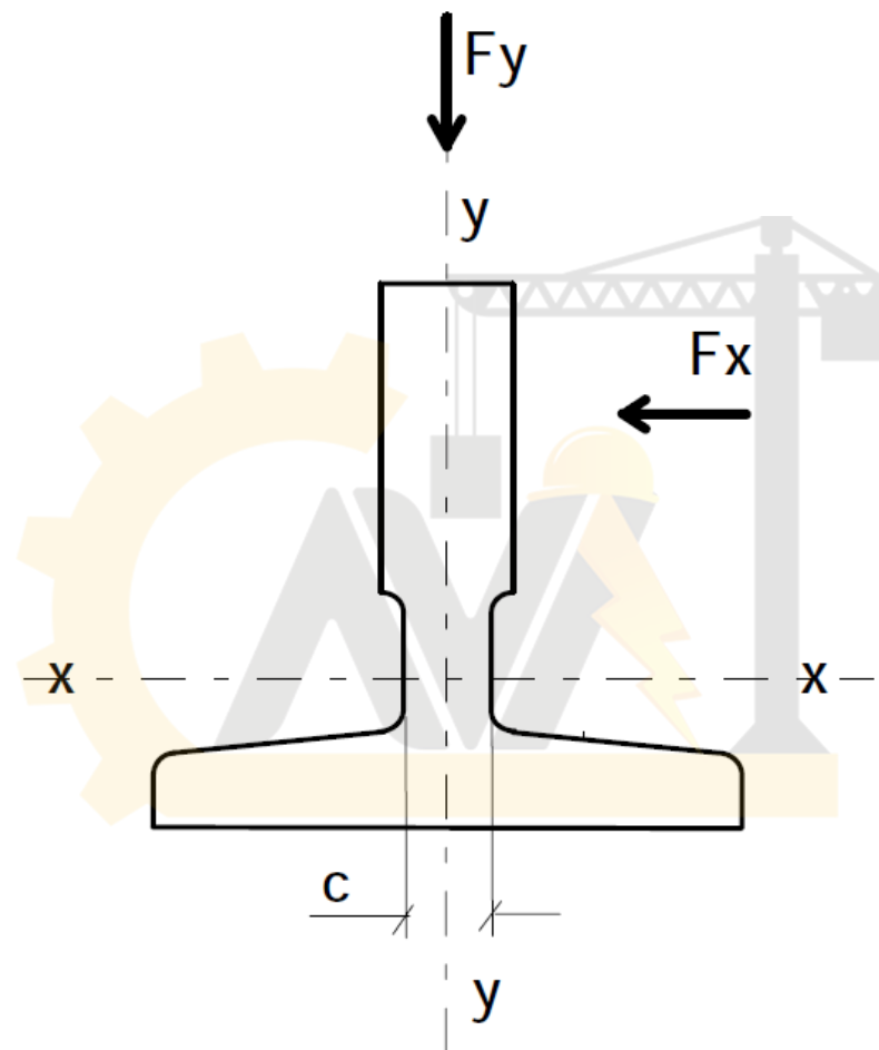
شکل چ-۱- محور ریل راهنما
