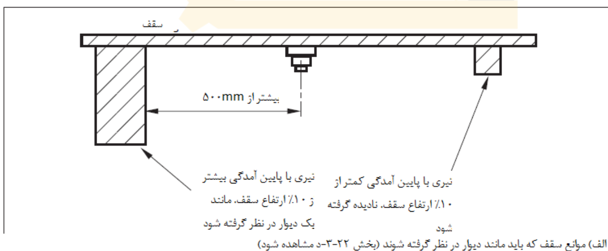
شکل ۱۰ - سقف
