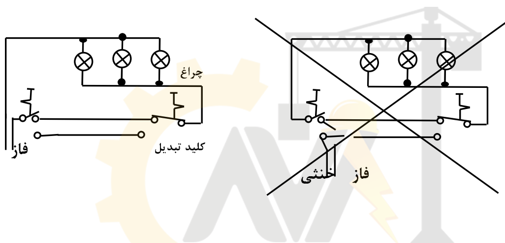
شکل ۳ نمایش روشهای صحیح و غلط سیم‌کشی با استفاده از کلیدهای تبدیل.
