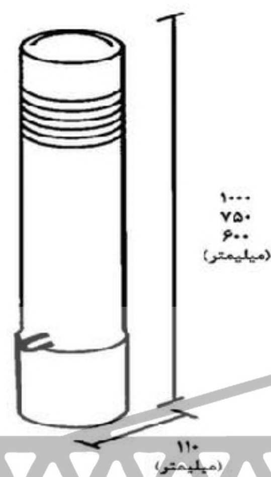
شکل ۴-۲۳-۴ ستون پارک‌بند در محیط پارکینگ
