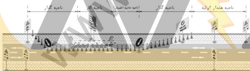
شکل پ ۲۳-۴-۳ محدوده حفاظت از عملیات کارگاهی در معبر با پیاده رو و یک خط
