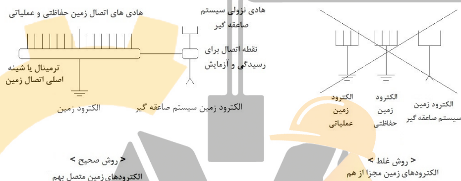
شکل پ ۳-۸-۲-۱ طرحواره نحوه اتصال الکترودهای زمین حفاظتی، عملیاتی و صاعقه‌گیر
