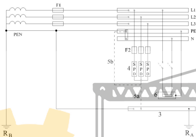
شکل ۱۳-۳-۱۶-۴:۱ طرحواره نصب برقگیر حفاظتی در شبکه توزیع سیستم نیروی TN (سه فاز)
