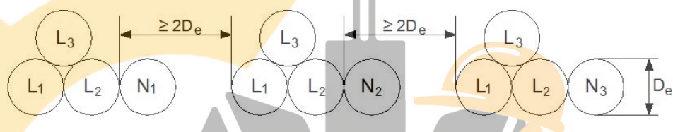
شکل ۶: ۱-۷-۱-۷-۱۳ آرایش مثلثی مخصوص برای ۹ رشته کابل تک رشته موازی (سه فاز)
