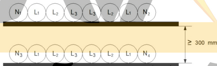
شکل ۸: ۱-۷-۱-۷-۱۳ آرایش چسبیده به هم در دو تراز به فاصله ۳۰ سانتی متر از هم برای ۱۲ رشته کابل تک رشته موازی (سه فاز)
