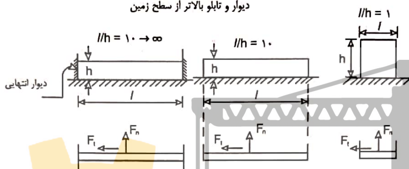
دیوار و تابلو روی سطح زمین
