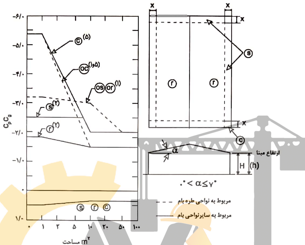
شکل ۶-۱۰-۶ ضرایب ترکیبی فشار و مکش خارجی C_p C_g برای طراحی پوشش‌ها و اجزاء بام (با زاویه شیب کمتر از 7^\circ درجه، با یا بدون طره)
