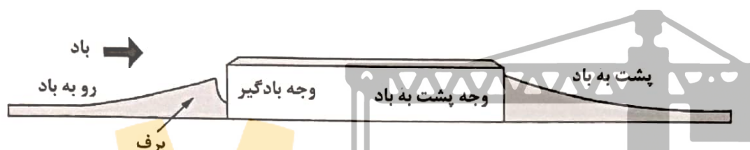
شکل ۶-۷-۷ نمایش وجه‌های رو به باد و پشت به باد
