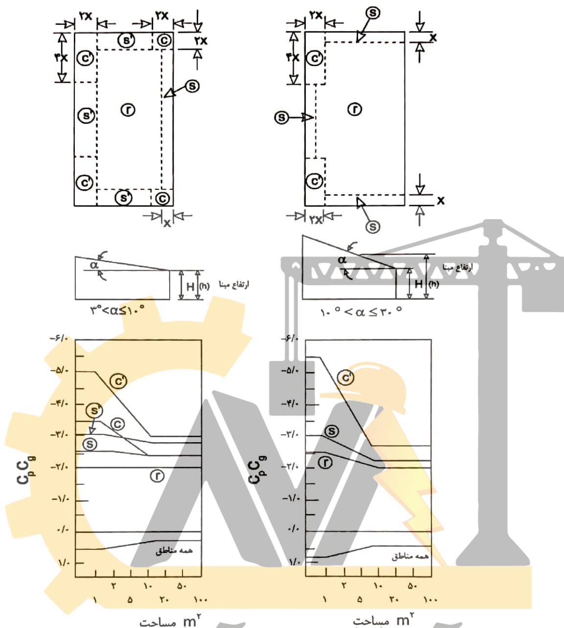
شکل ۶-۱۰-۹ ضرایب ترکیبی فشار و مکش خارجی C_p C_g برای طراحی پوشش‌ها و اجزاء بام‌های شیب‌دار یک‌طرفه
