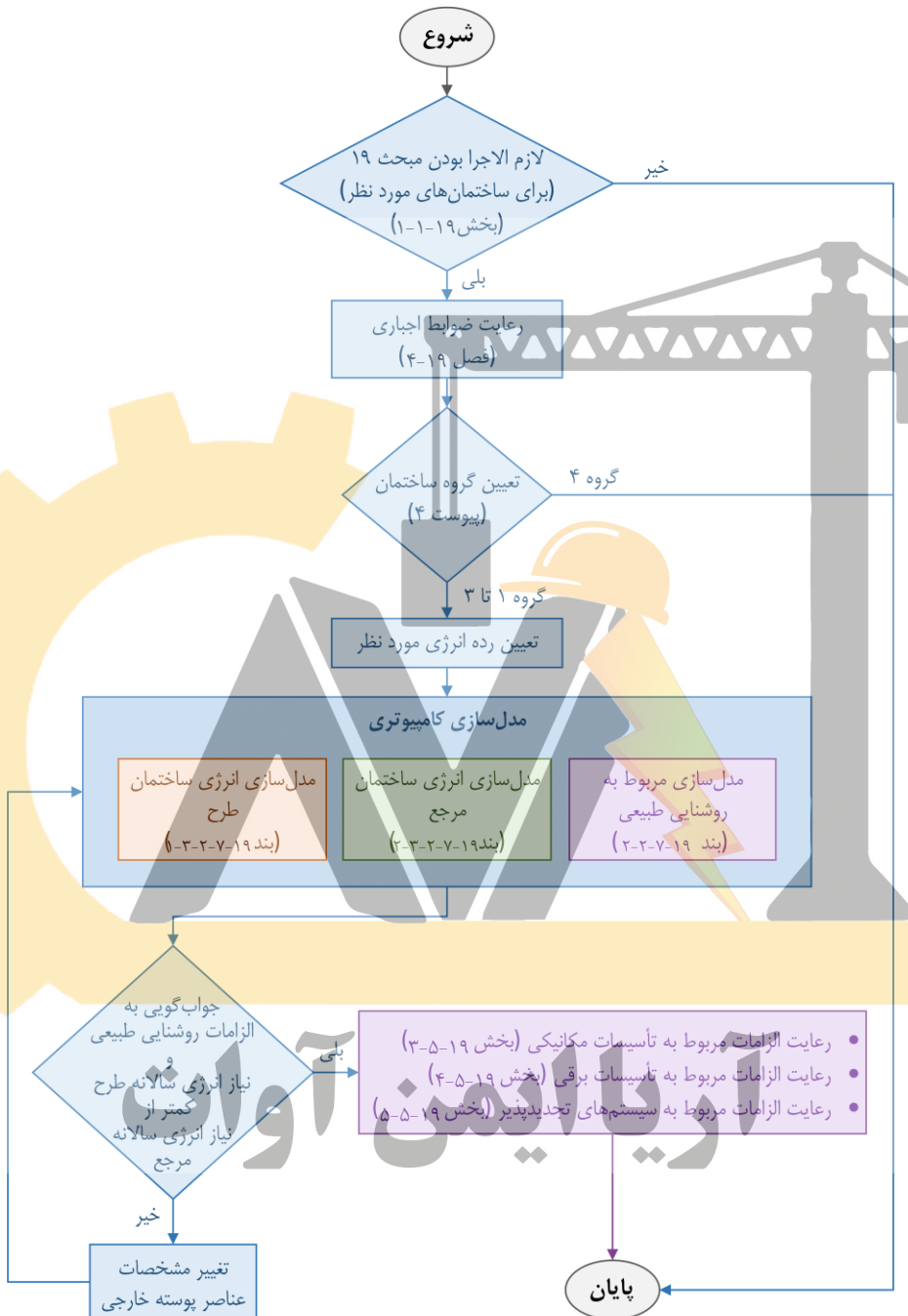
شکل ۷-۱۹-۱ نمودار گردش مراحل روش نیاز انرژی
