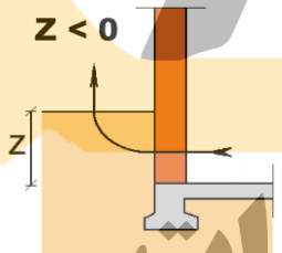
شکل پ ۱۱-۶ انتقال حرارت خطی ی دیوار مجاور خاک
