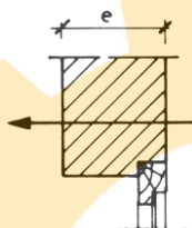
شکل پ ۱۱-۱۳ بازشوهای همباد داخل در دیوارهای بدون عایق حرارتی یا با عایق همگن
