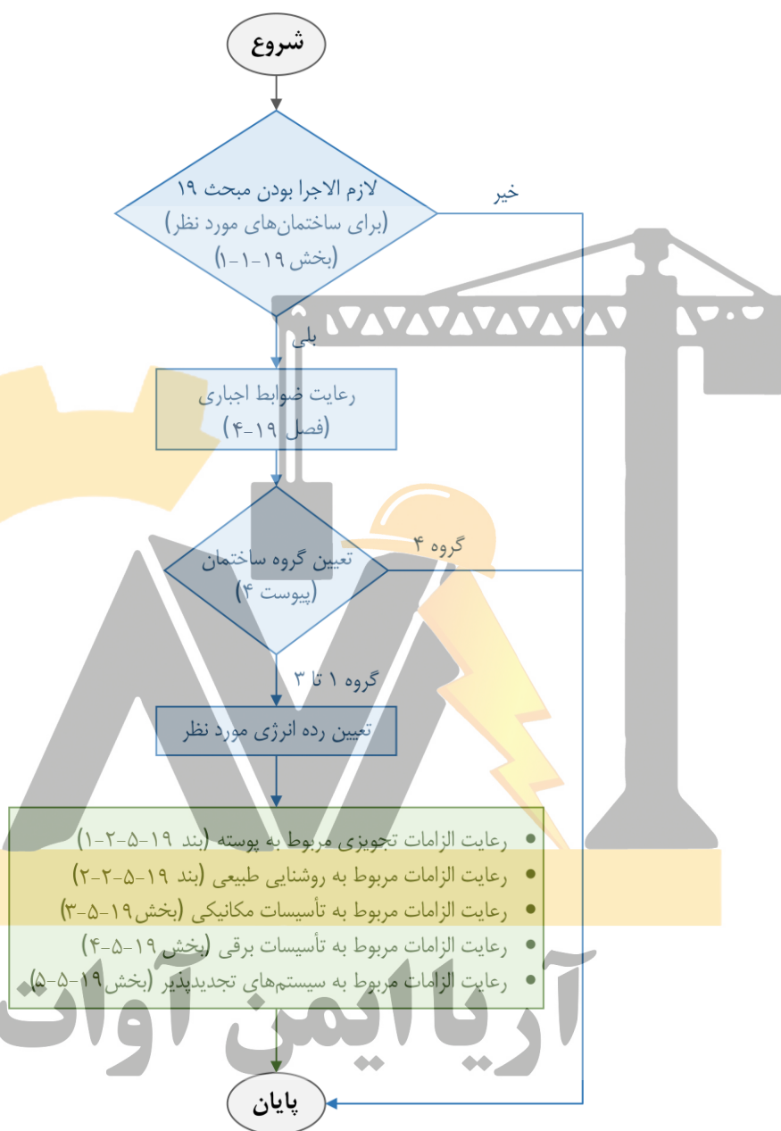
شکل ۵-۱۹-۱ نمودار گردش مراحل روش تجویزی
