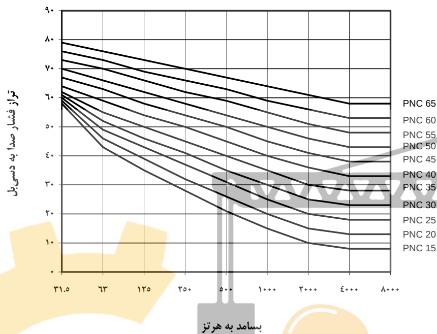
شکل ۱۸-۳-۵: نمودارهای پرسنج ترجیحی نوفه PNC
