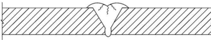
شکل ۱۷-۶-۴ ترک‌های ستاره‌ای در سطح جوش
