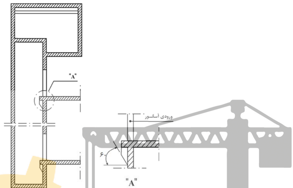
شکل ۲-۱۵-۳-۳-۳ سطح داخلی دیواره چاه در سمت ورودی طبقات.
